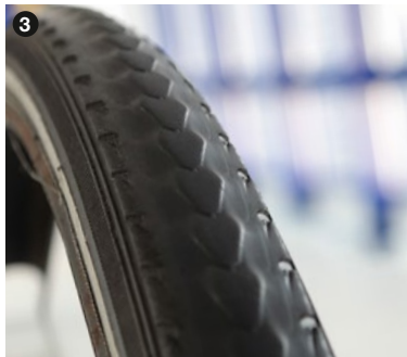
Abriebspuren
